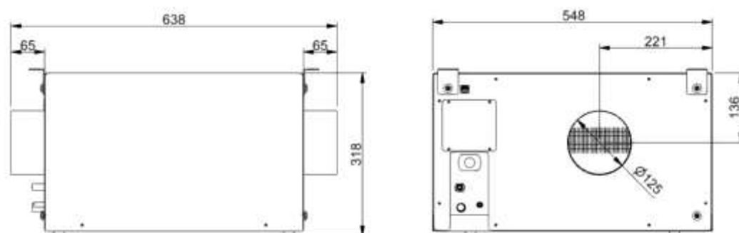
Unité intérieure
